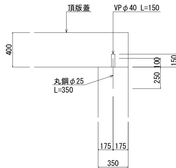
ズレ止め詳細図
