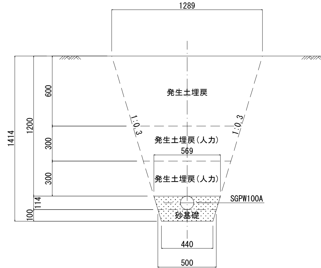
管埋設標準断面図 S=1:20 (SGPW100A)
