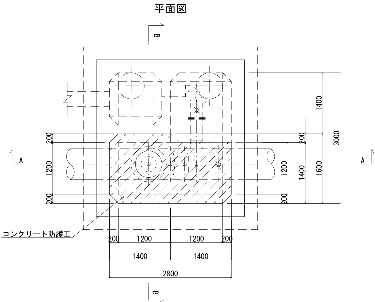
コンクリート防護工
