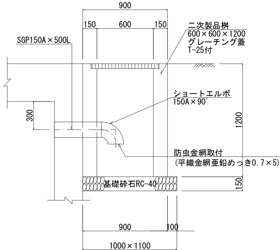
A-A断面
