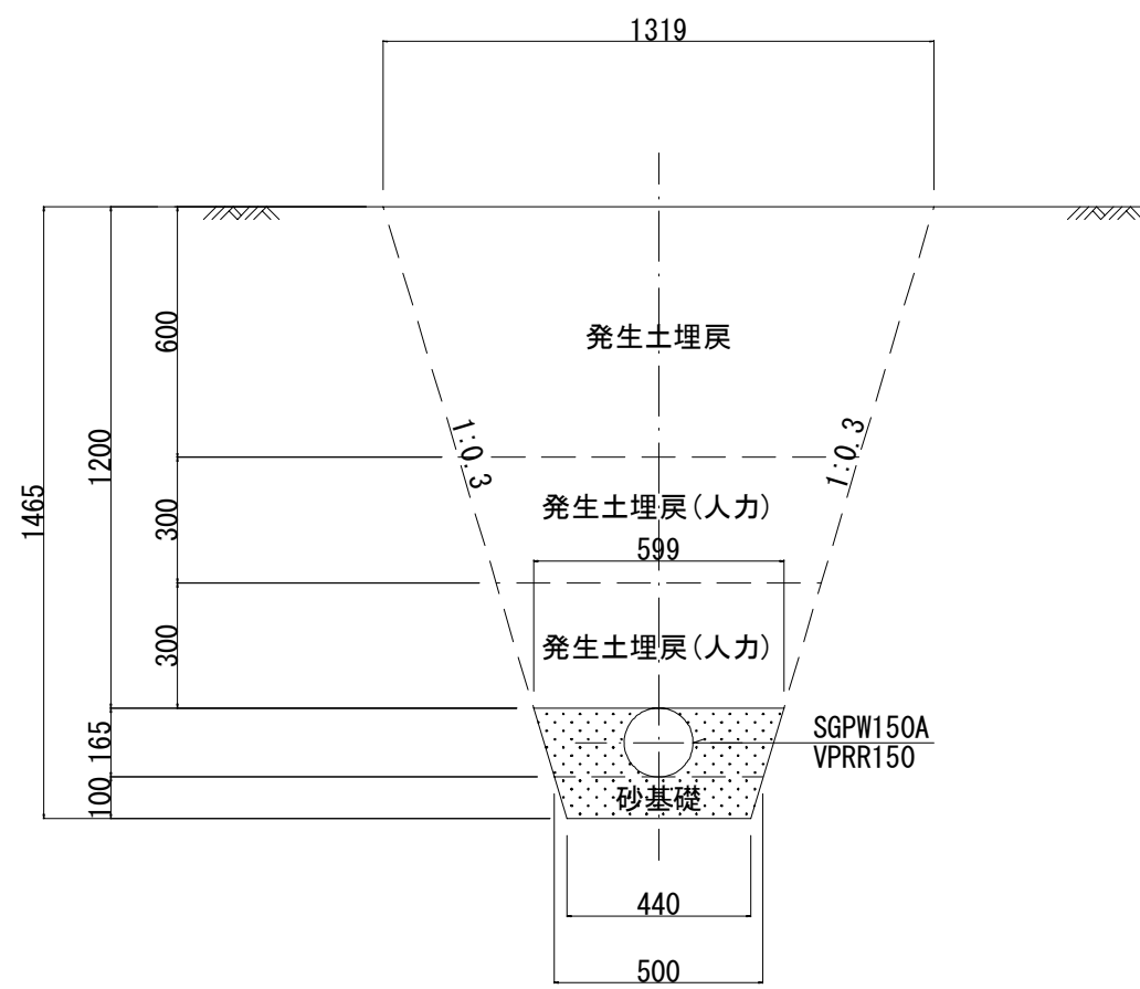
管埋設標準断面図 S=1:20 (SGPW150A, VPRR150)
