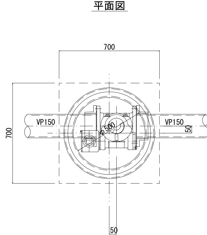
手動式バタフライ弁 S=1:15
