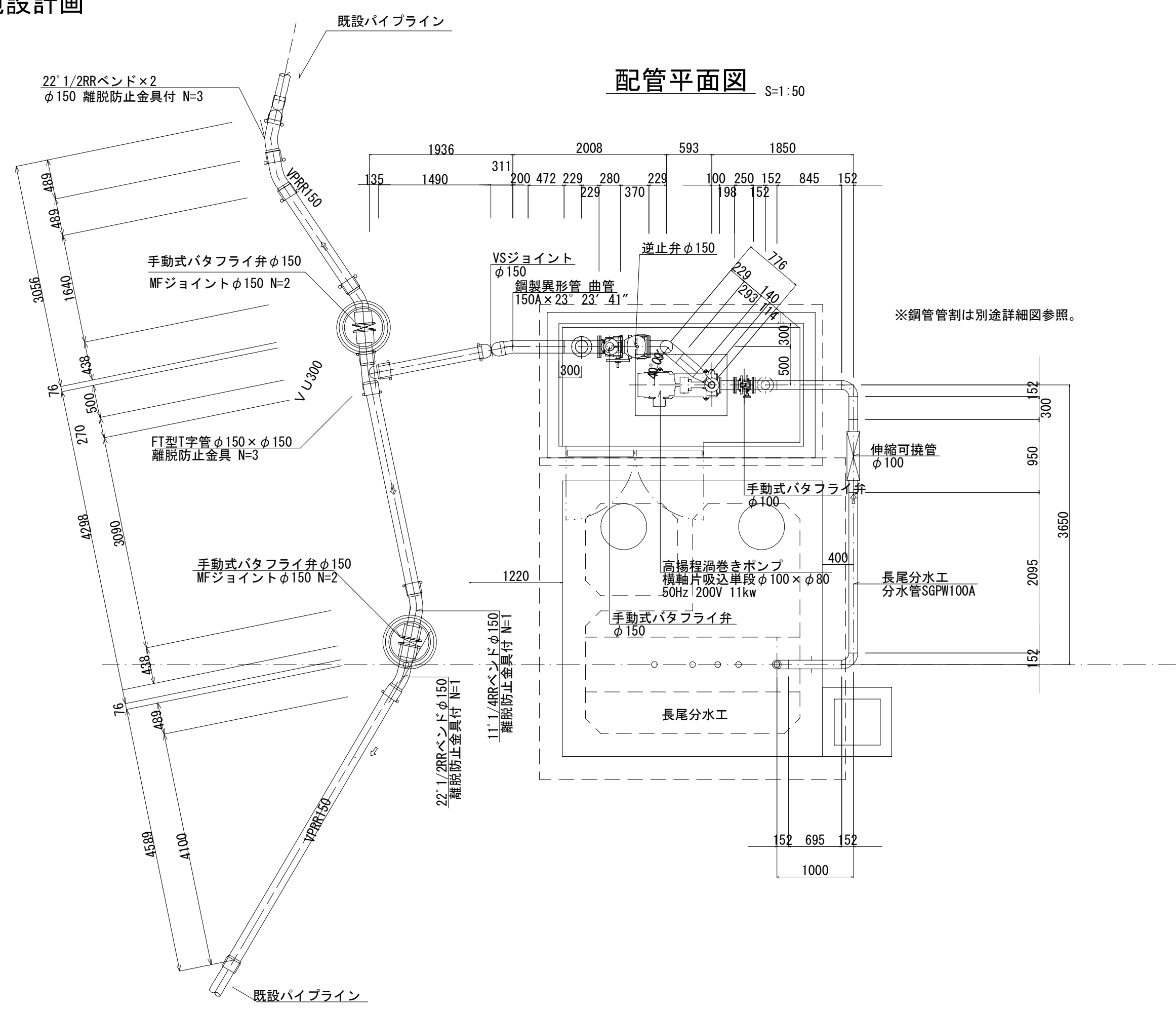
ポンプ基礎詳細図 S=1:25
