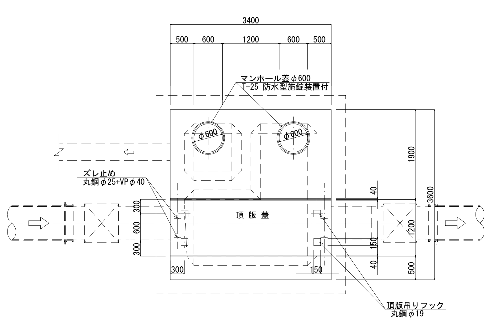
頂版平面図
