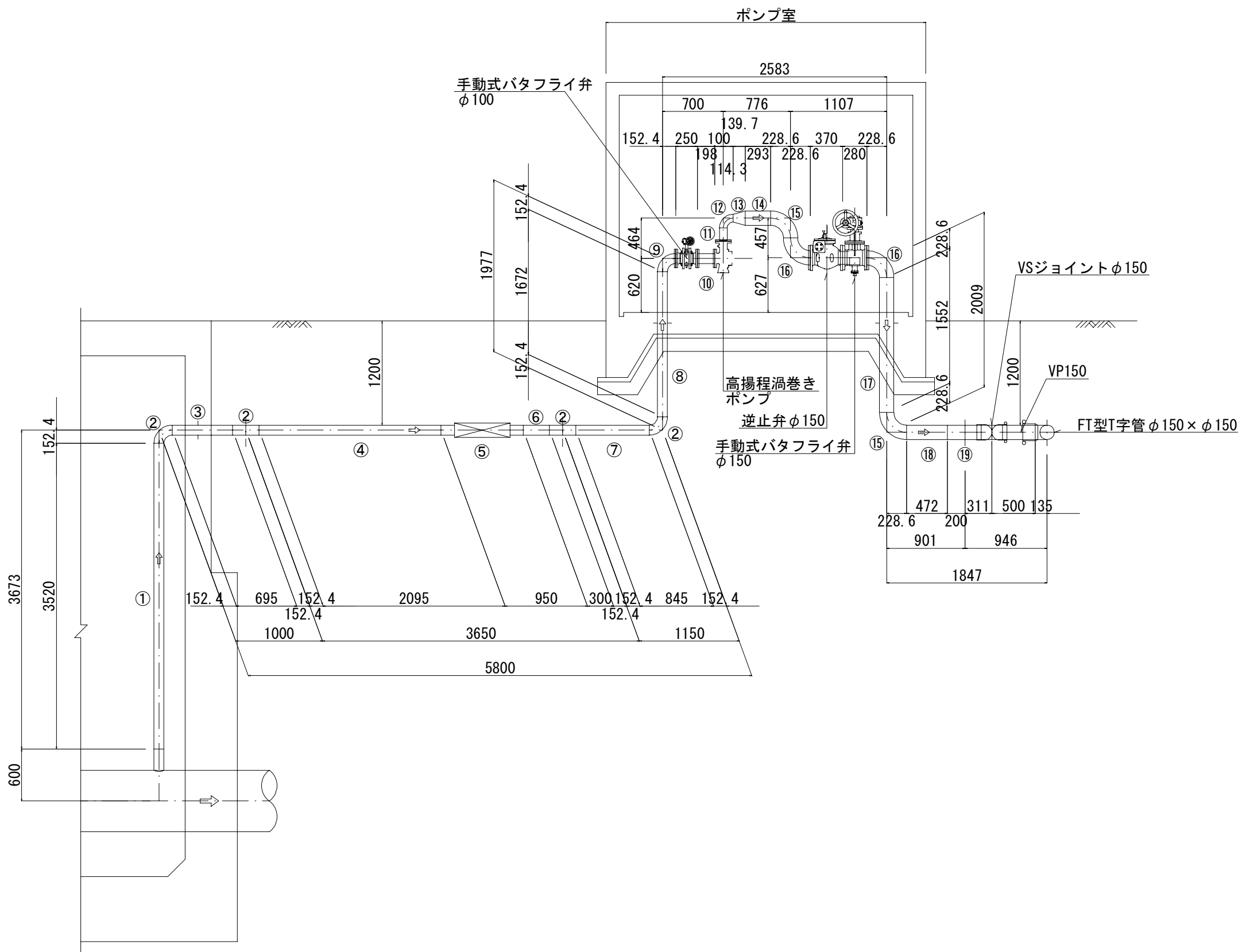
鋼管管割詳細図 S=1:50
