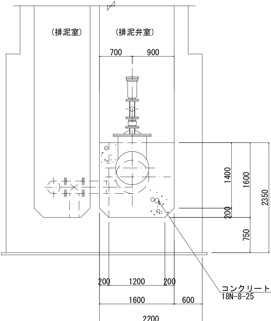
B-B断面
