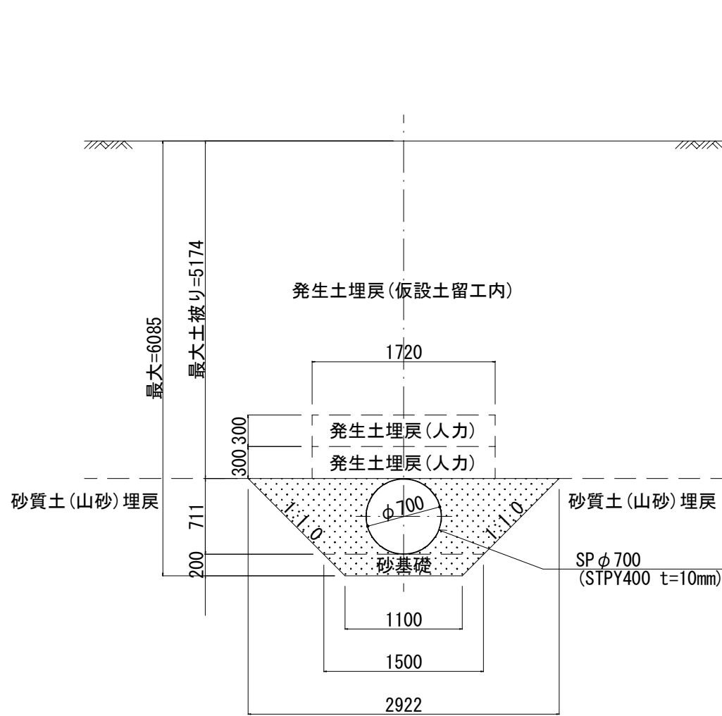
管理設標準断面図
