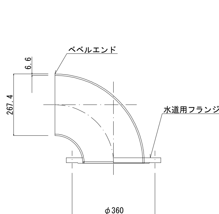
②90°エルボ(シヨート, FSGP) 250A
