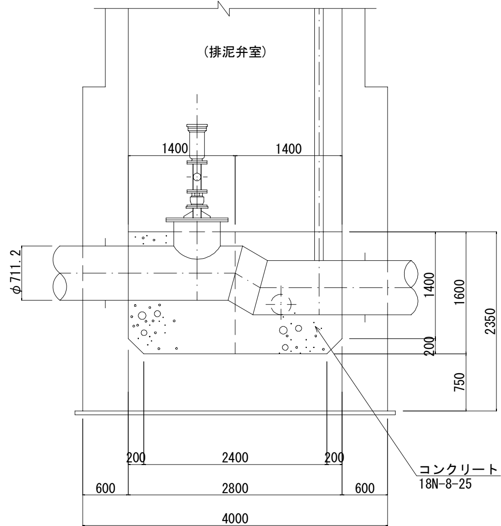
A-A断面
