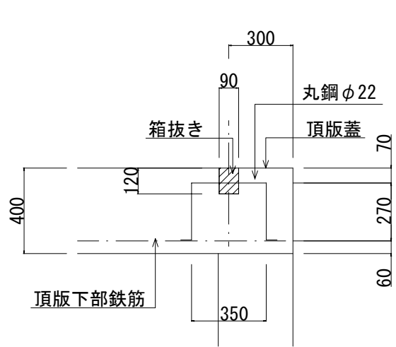
頂版吊りフック詳細図
