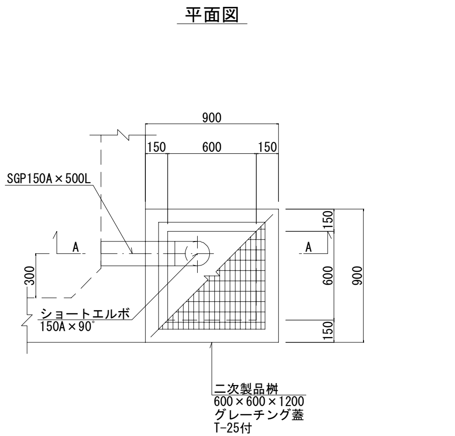
通気柵口600
