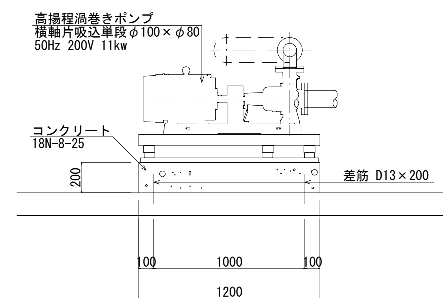
断面図
