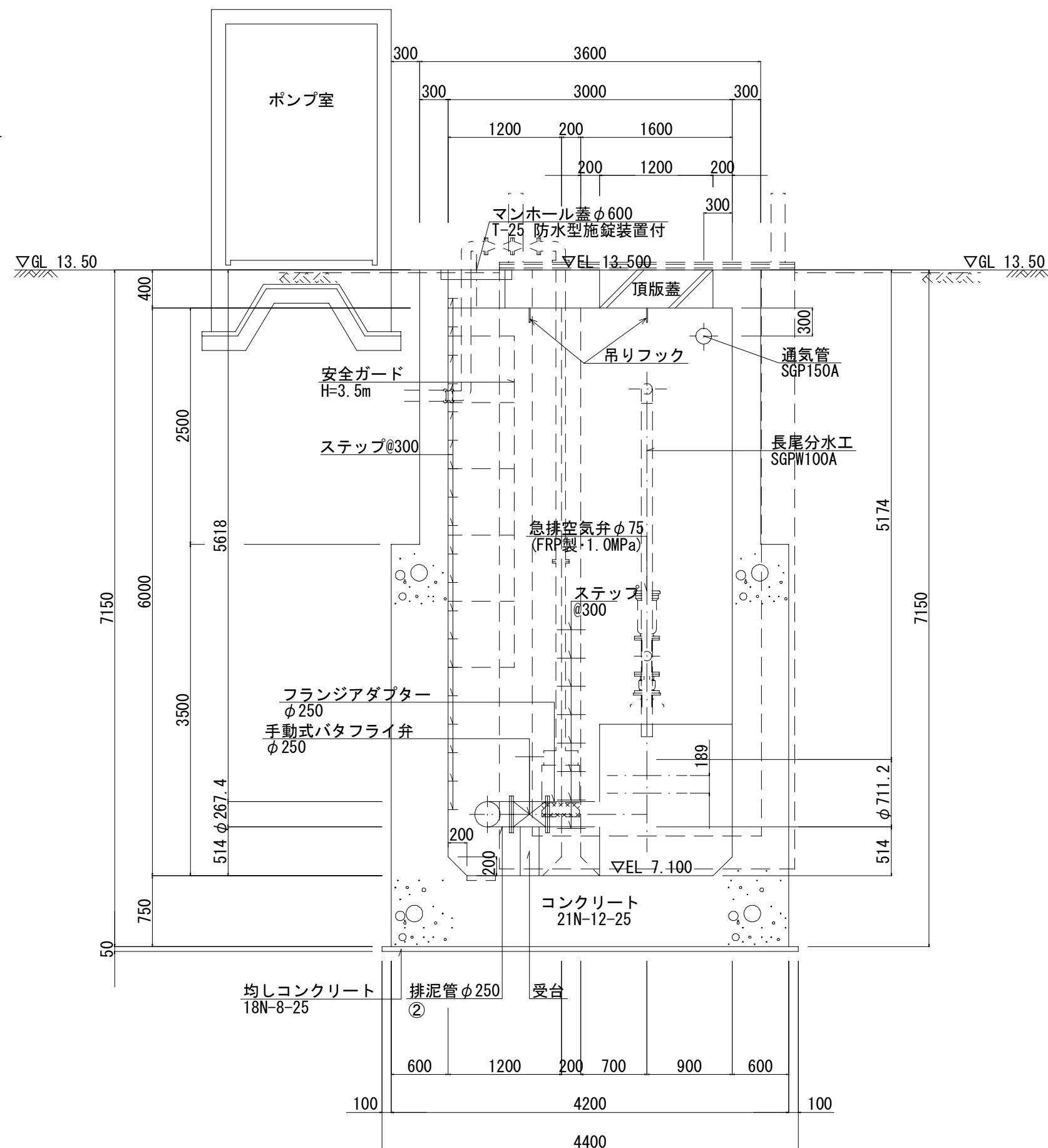
横断面図
