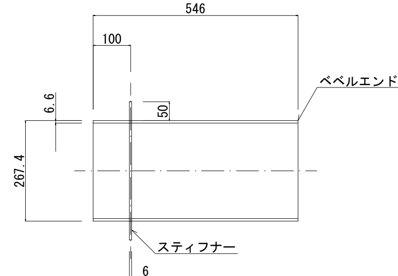
①スティフナー付短管 SGPW 250A x L546
