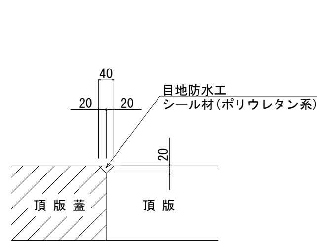
目地防水工詳細図
