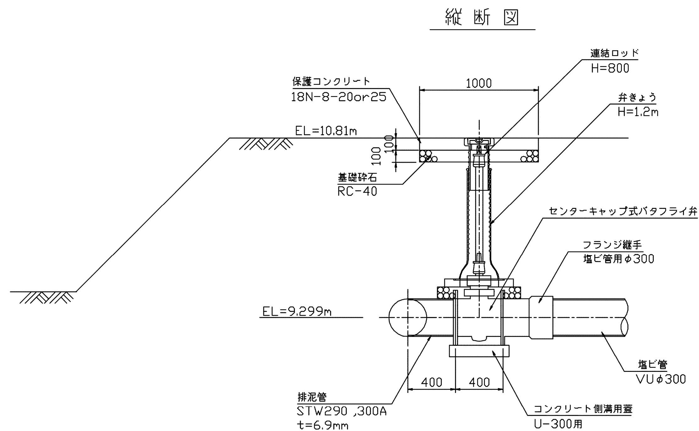
排泥弁構造図 S=1:20
