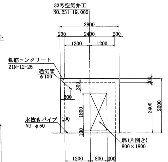
建屋正面図 S=1:50
