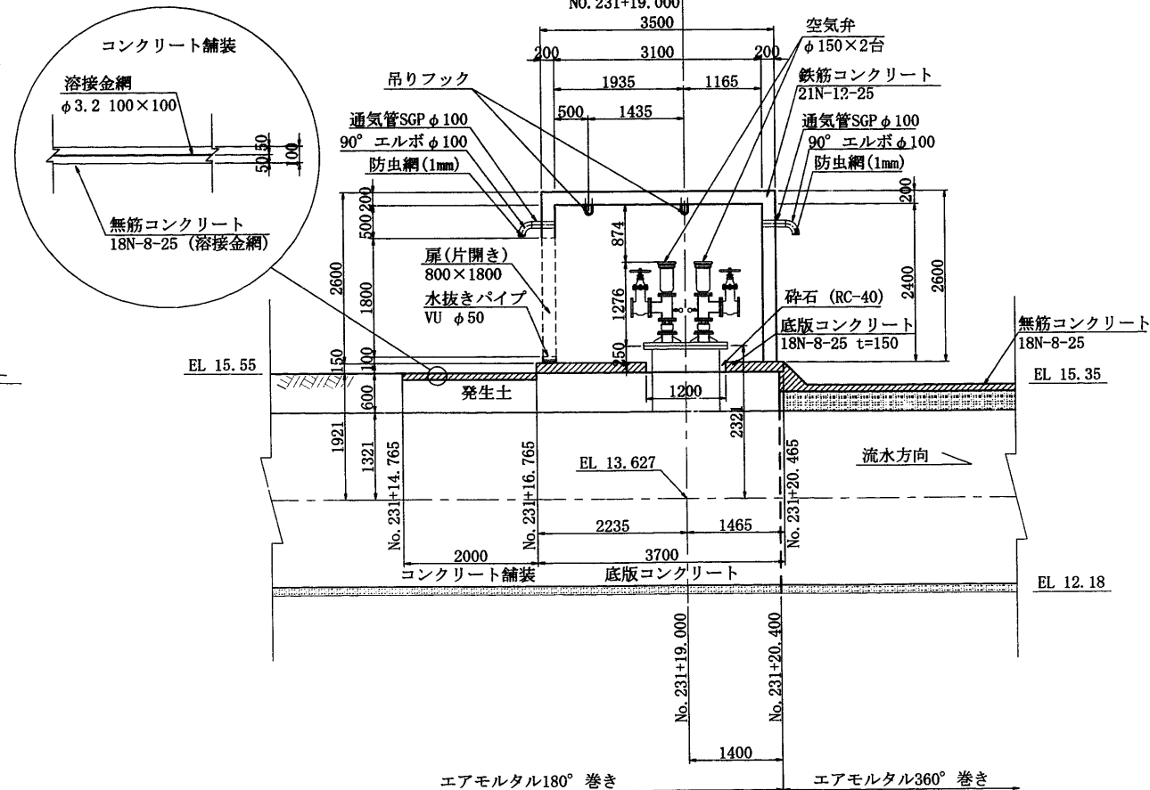
縦断図 S=1:50
