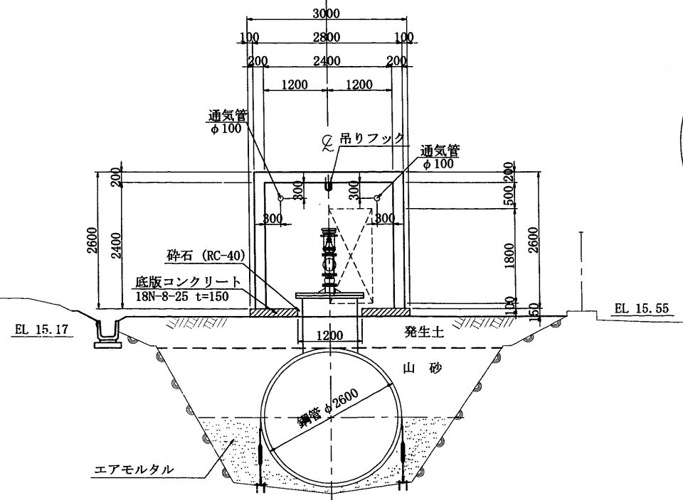
A-A S=1:50 33号空気弁工 NO. 231+19.000
