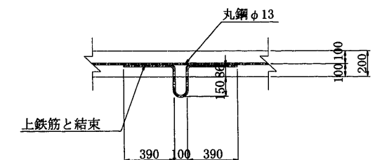
吊りフック詳細図 S=1:20
