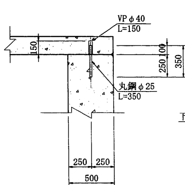
ずれ止め工詳細図 S=1:20
