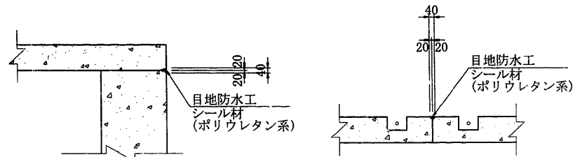
目地防水工詳細図 S=1:20
