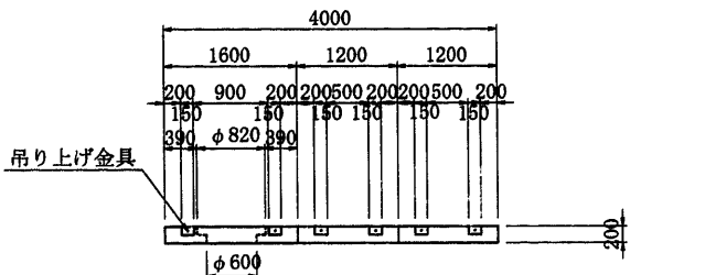
床版断面図 S=1:50
