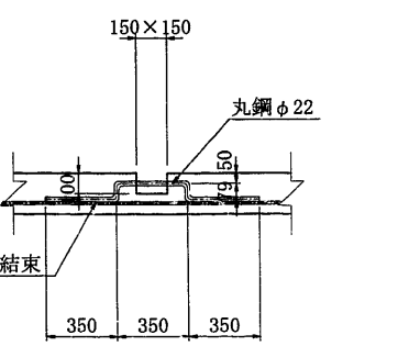
吊り上げ金具詳細図 S=1:20
