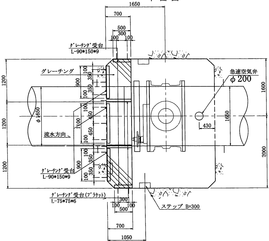
平面図
