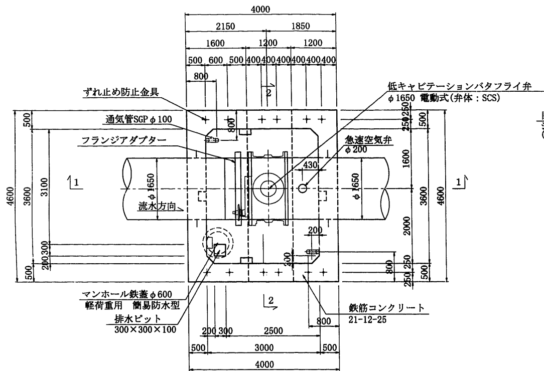
平面図 S=1:50
