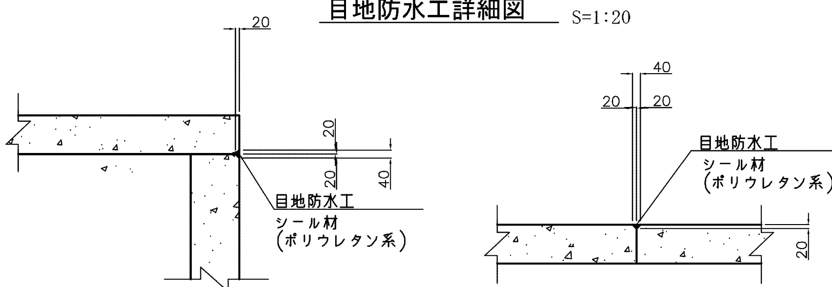
目地防水工詳細図
