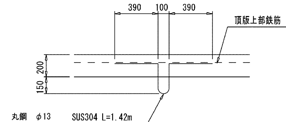
吊りフック詳細図
