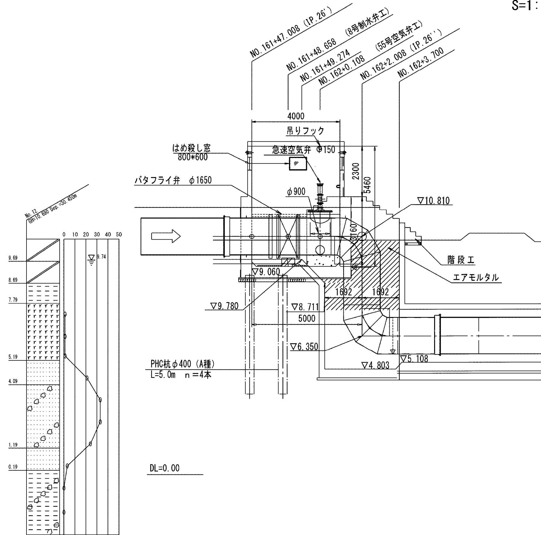
縦断面図
