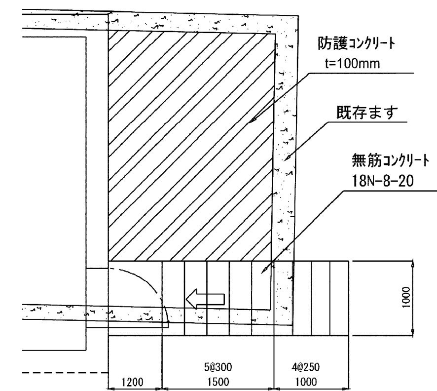
断面図
