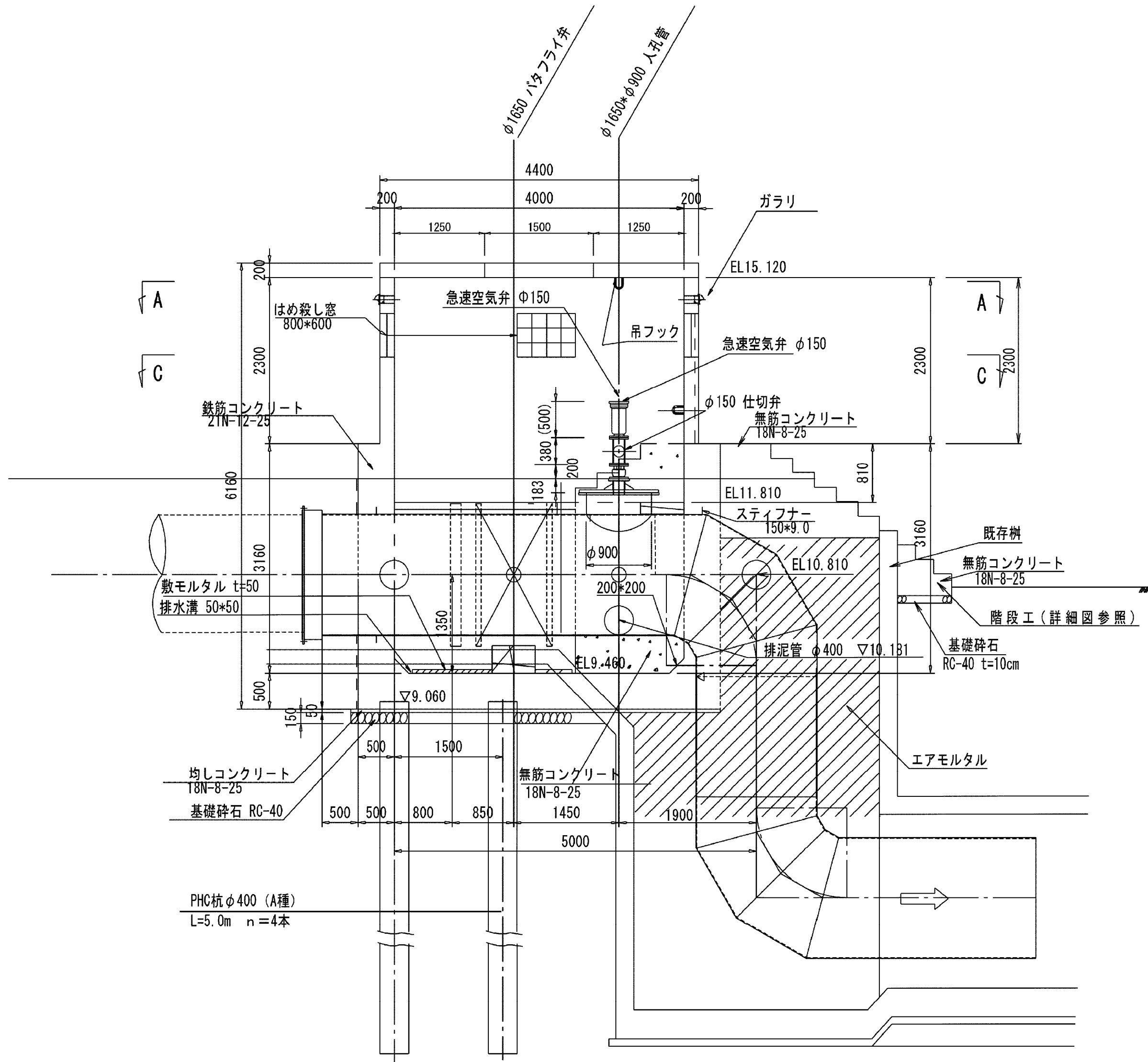
B - B
