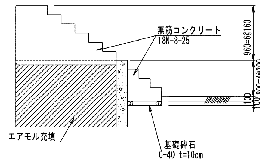
断面図
