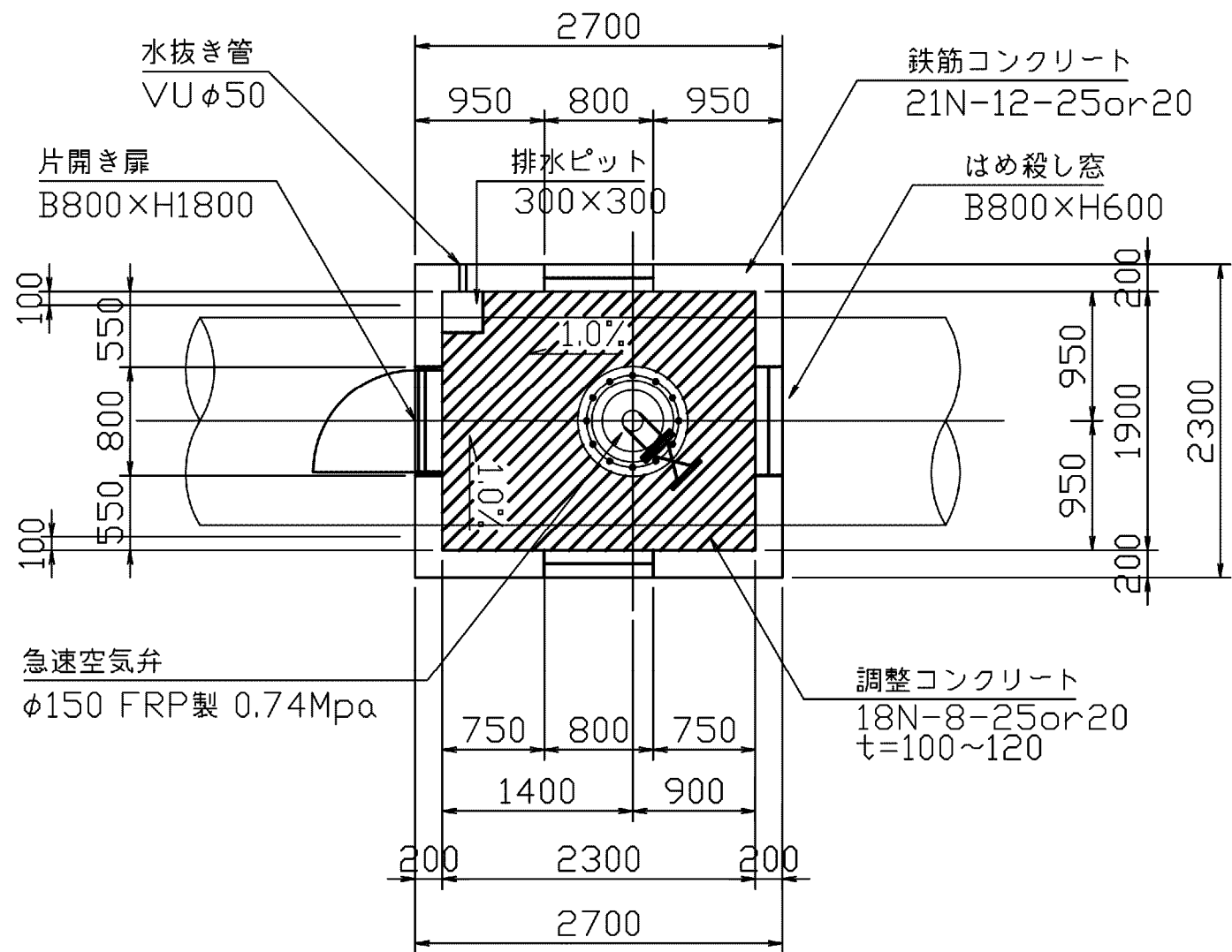
平断面図
