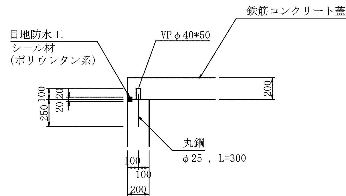
目地防水工詳細図
