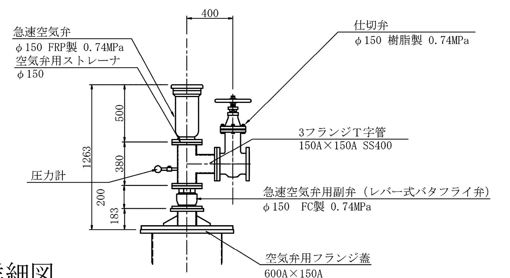
空気弁詳細図
