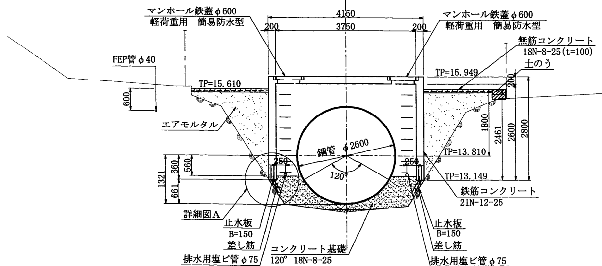
排水用塩ビ管 \phi 75 200 250 エアモルタル 差し筋 D13 L=780 止水板 B=150 コンクリート基礎 120° 18N-8-25
