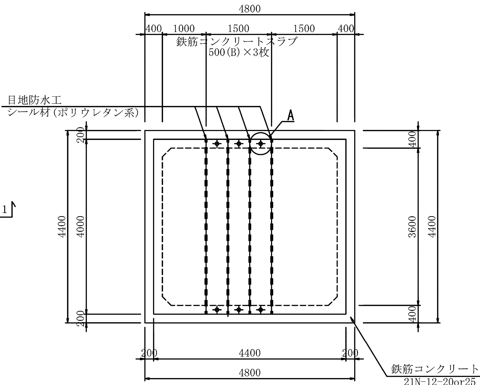
床版断面図 S=1:50
