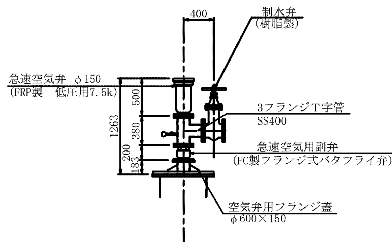
空気弁詳細図
