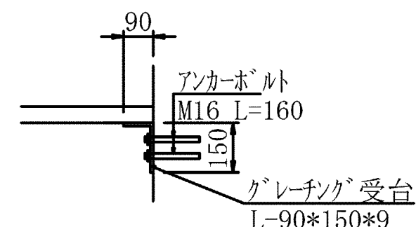
グレーチング受台
