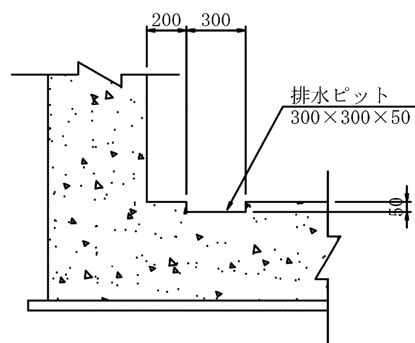
断面図
