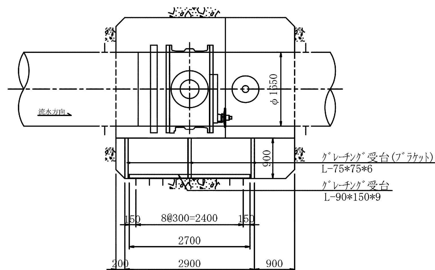
ブラケット
