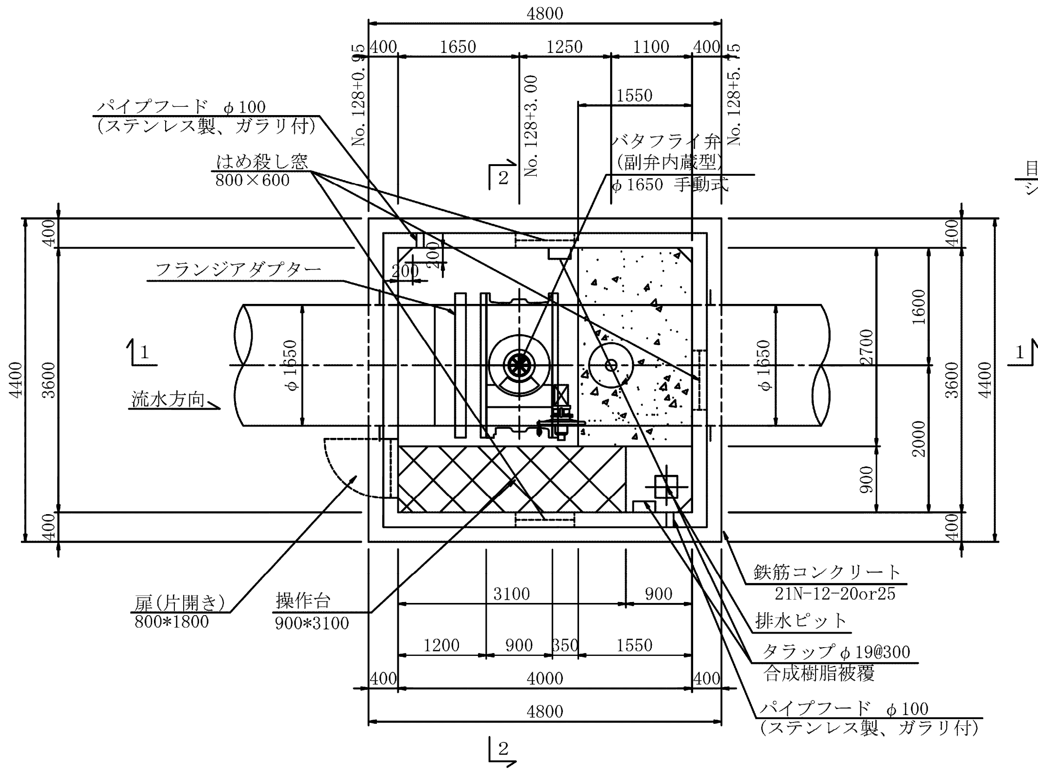
平面図 S=1:50
