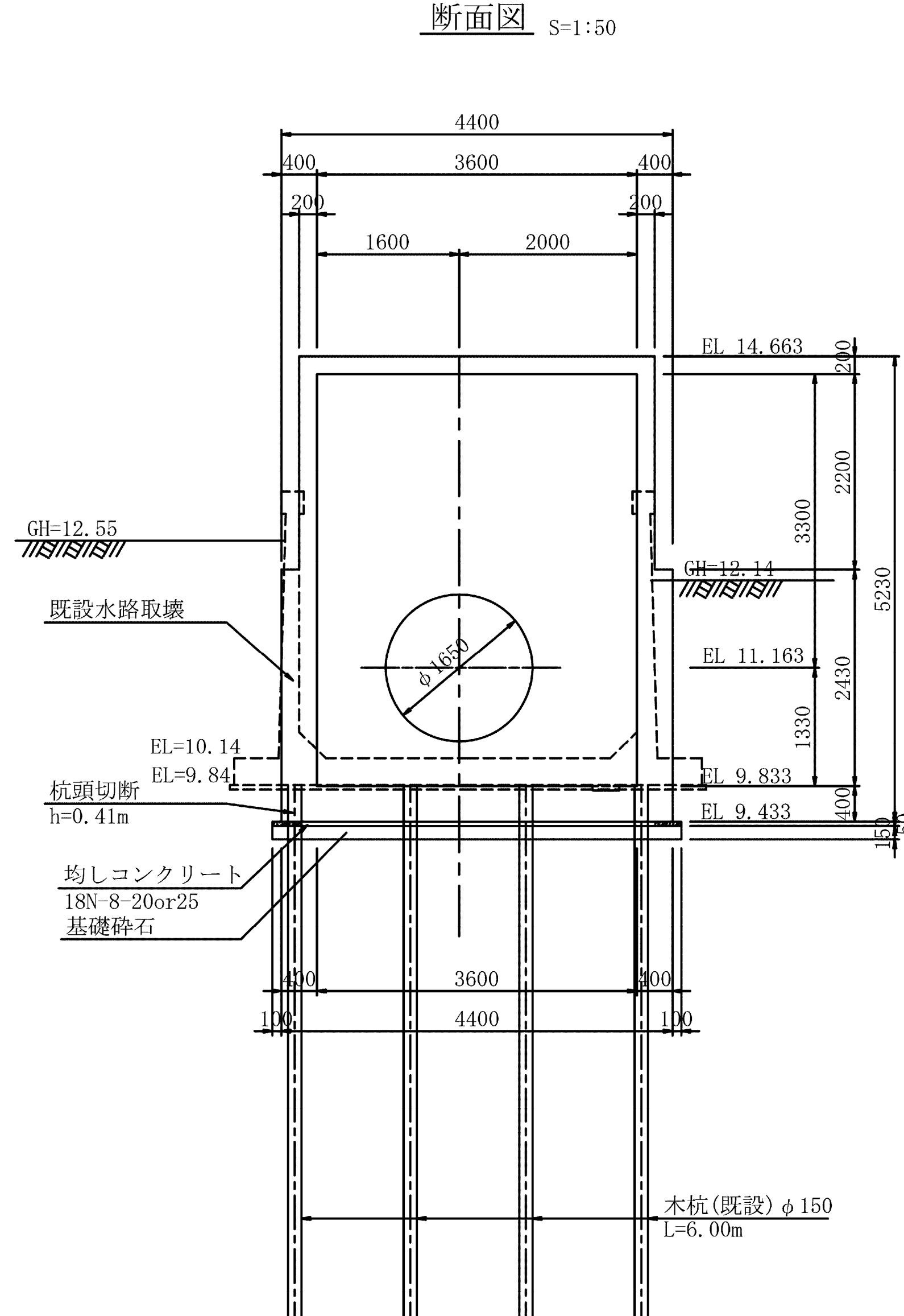
断面図
