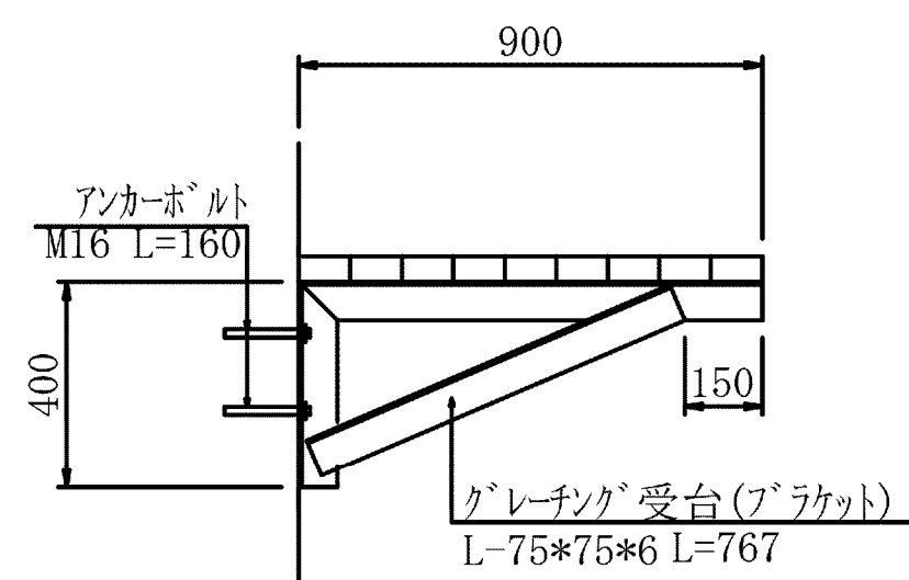
ブラケット
