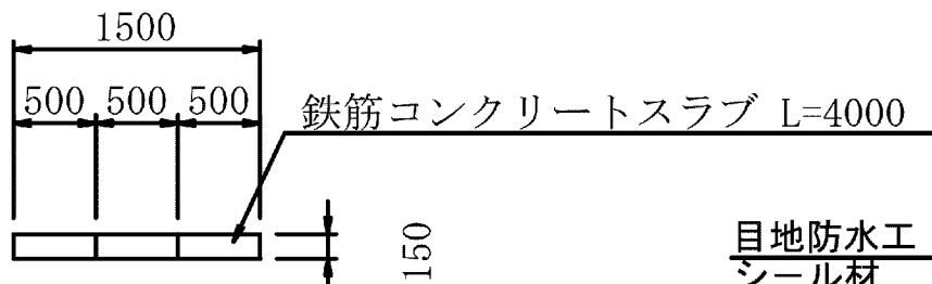
床版断面図 S=1:50
