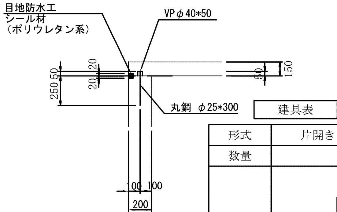
A 部詳細 S=1:20
