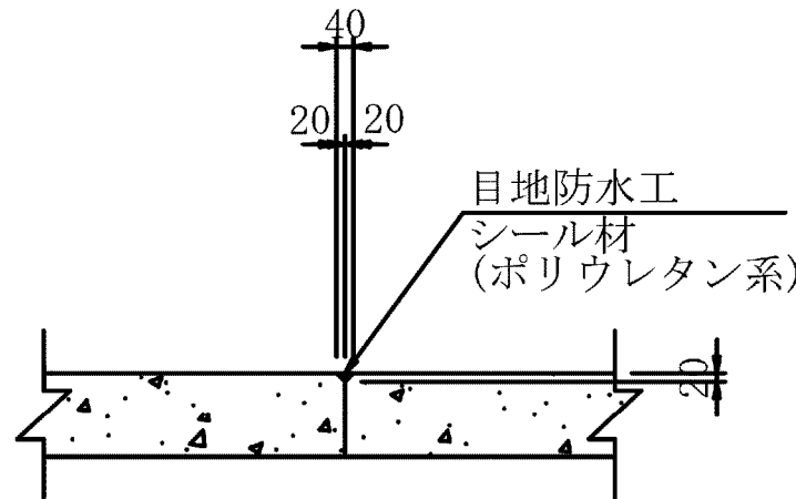
目地防水工詳細図 S=1:20
