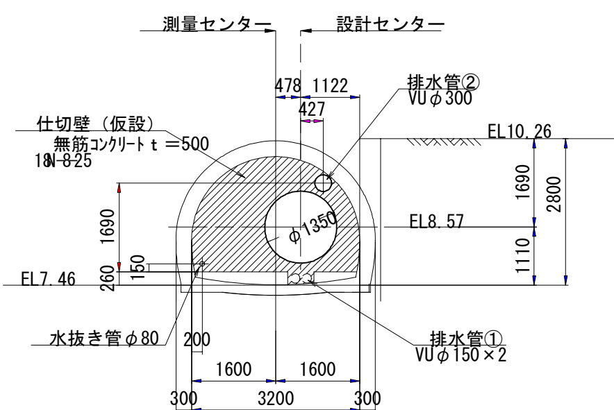
A-A断面
