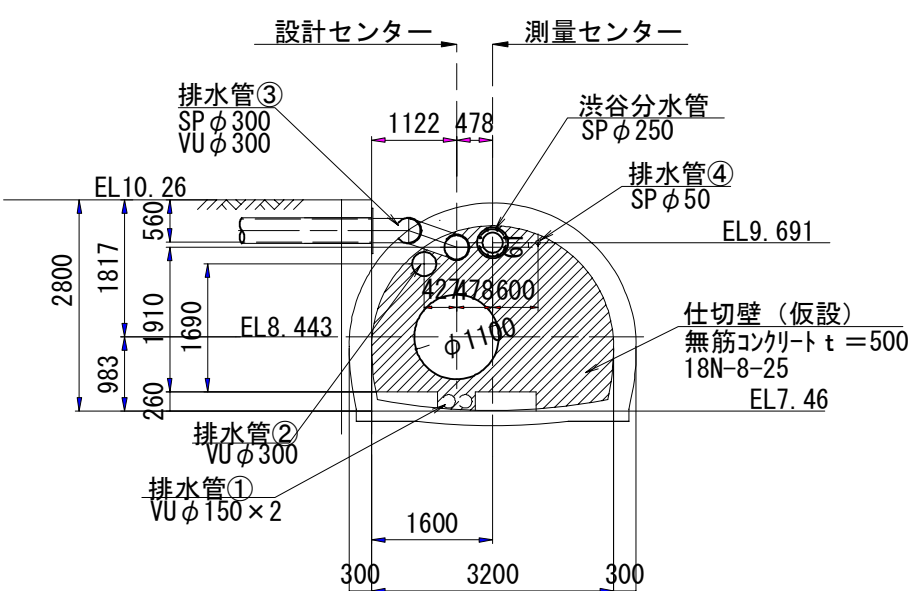
B-B断面
