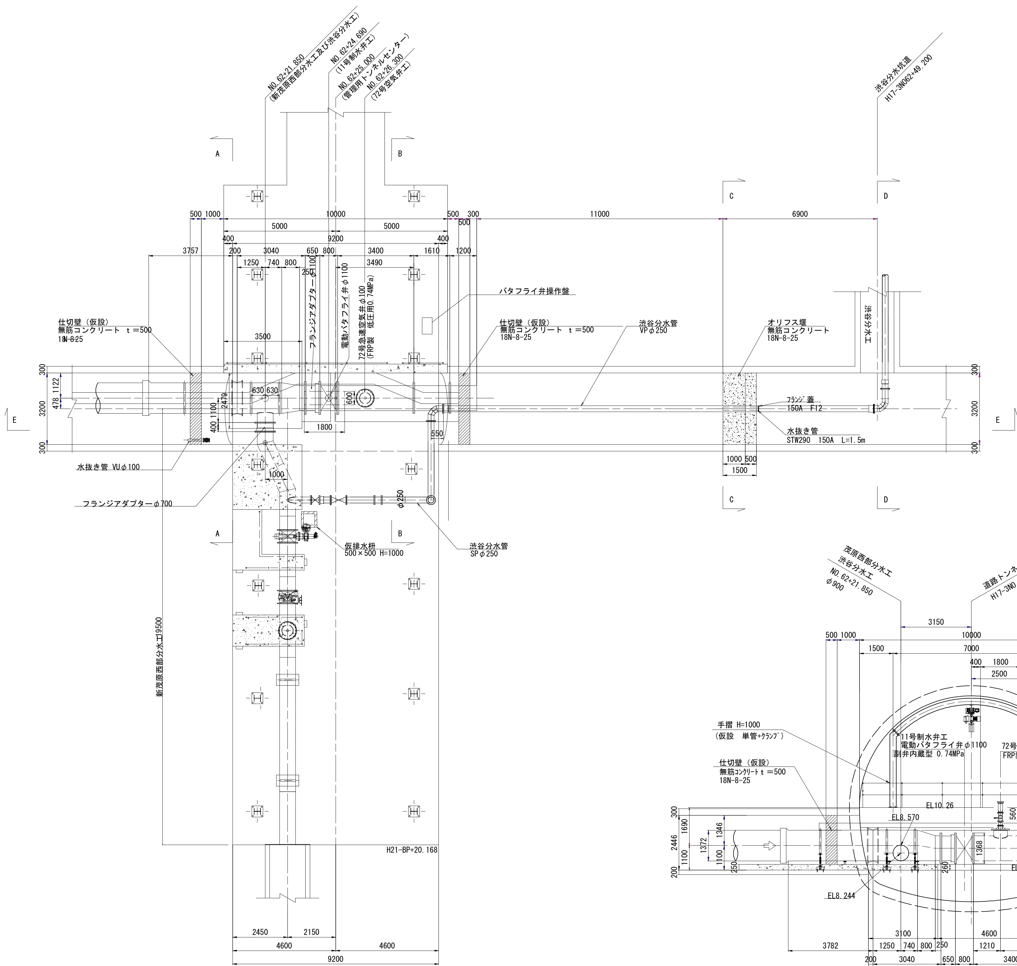
平面図
