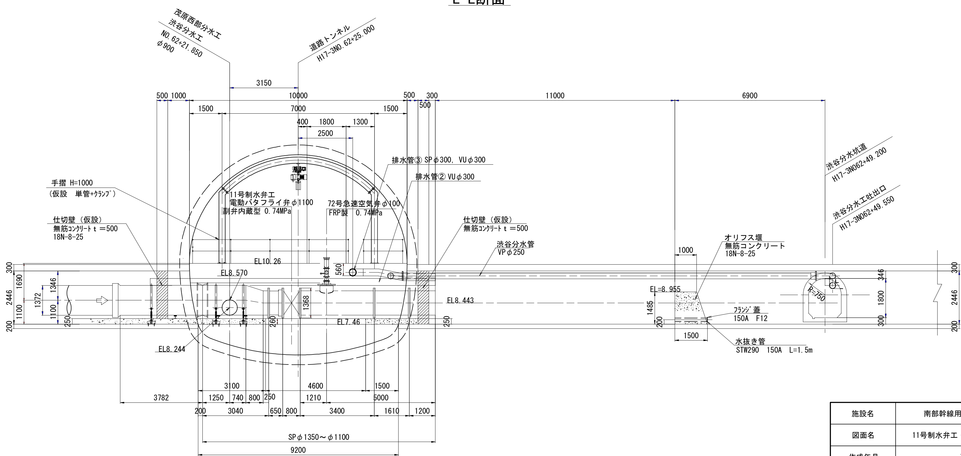
E-E断面
