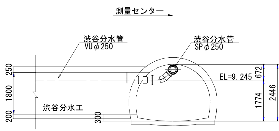
D-D断面
