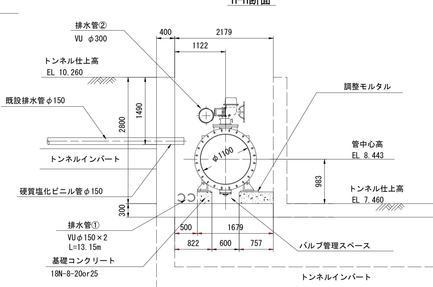
H-H断面
