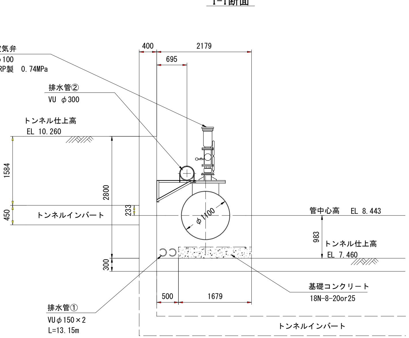
I-I断面
