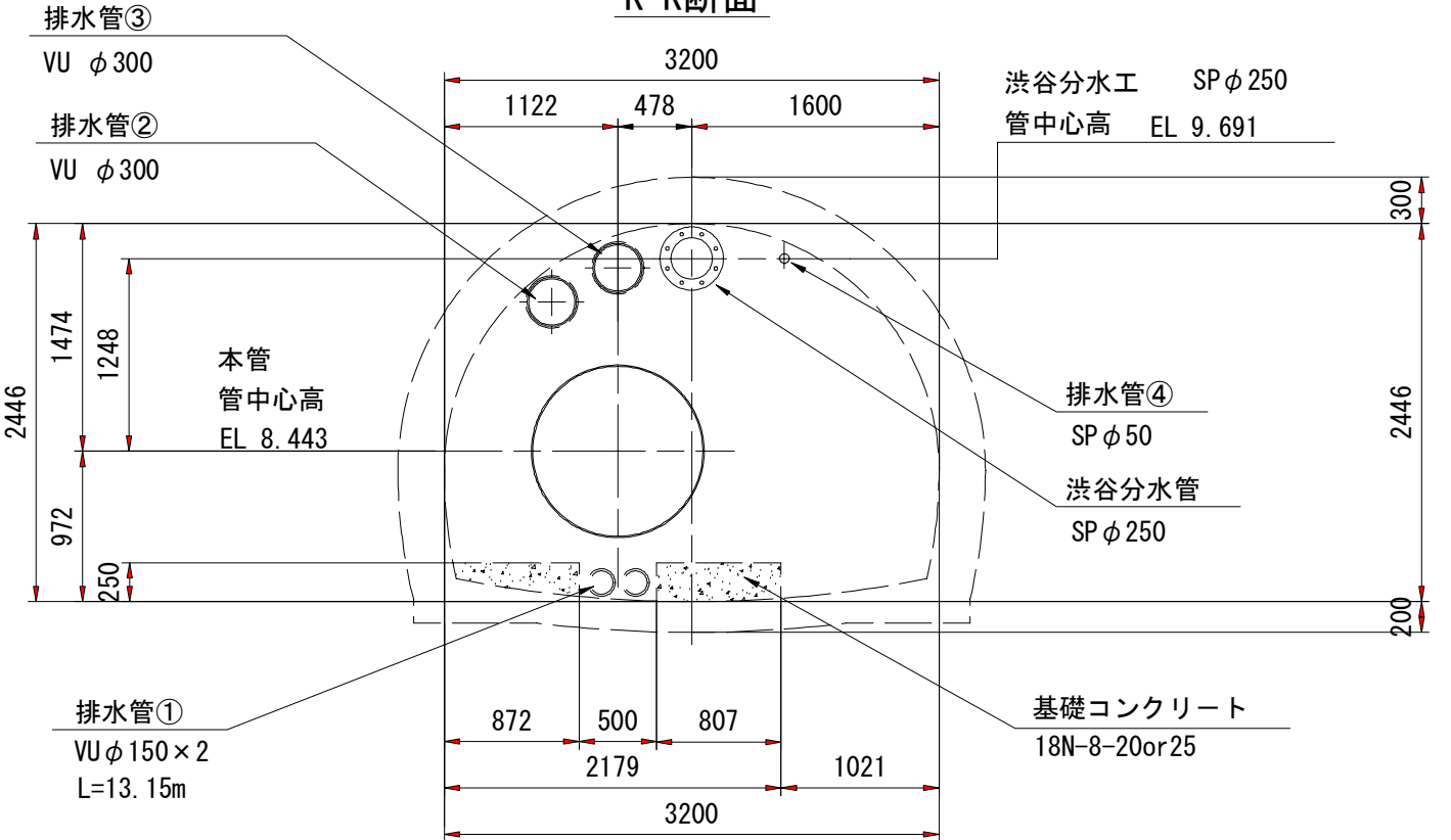
K-K断面
