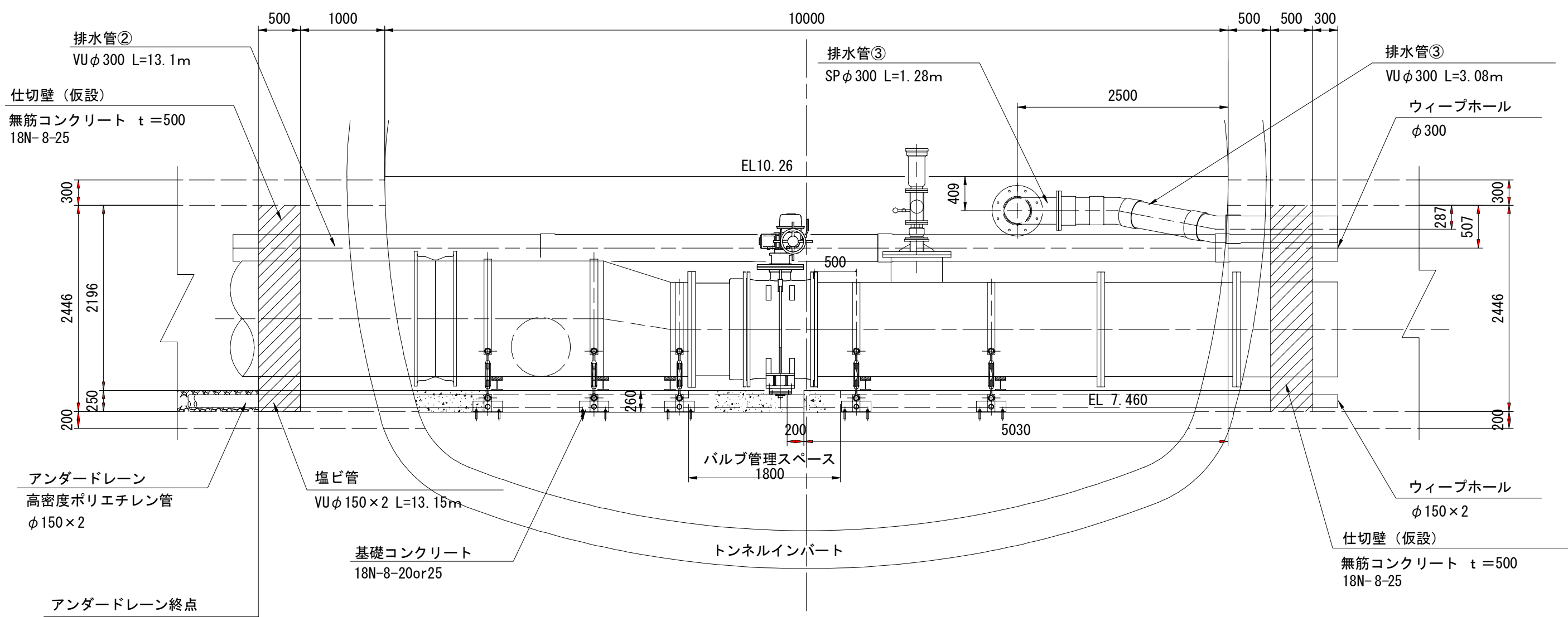
F-F断面
