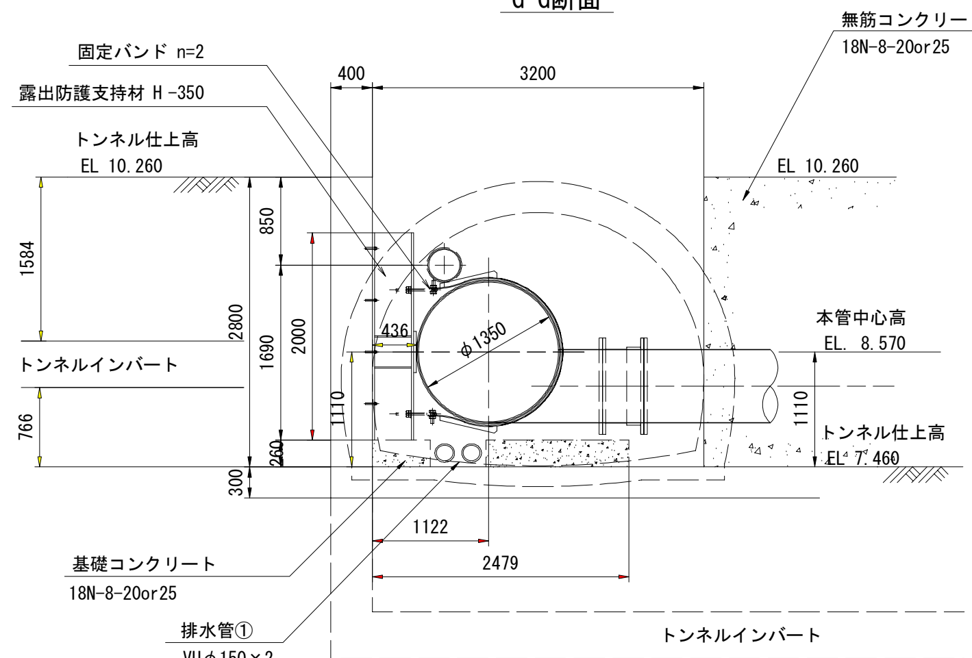
G-G断面
