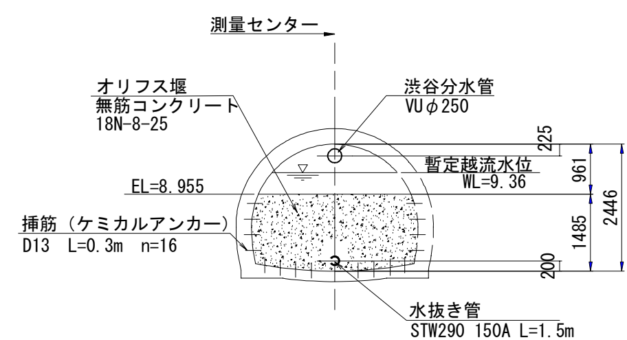
C-C断面
