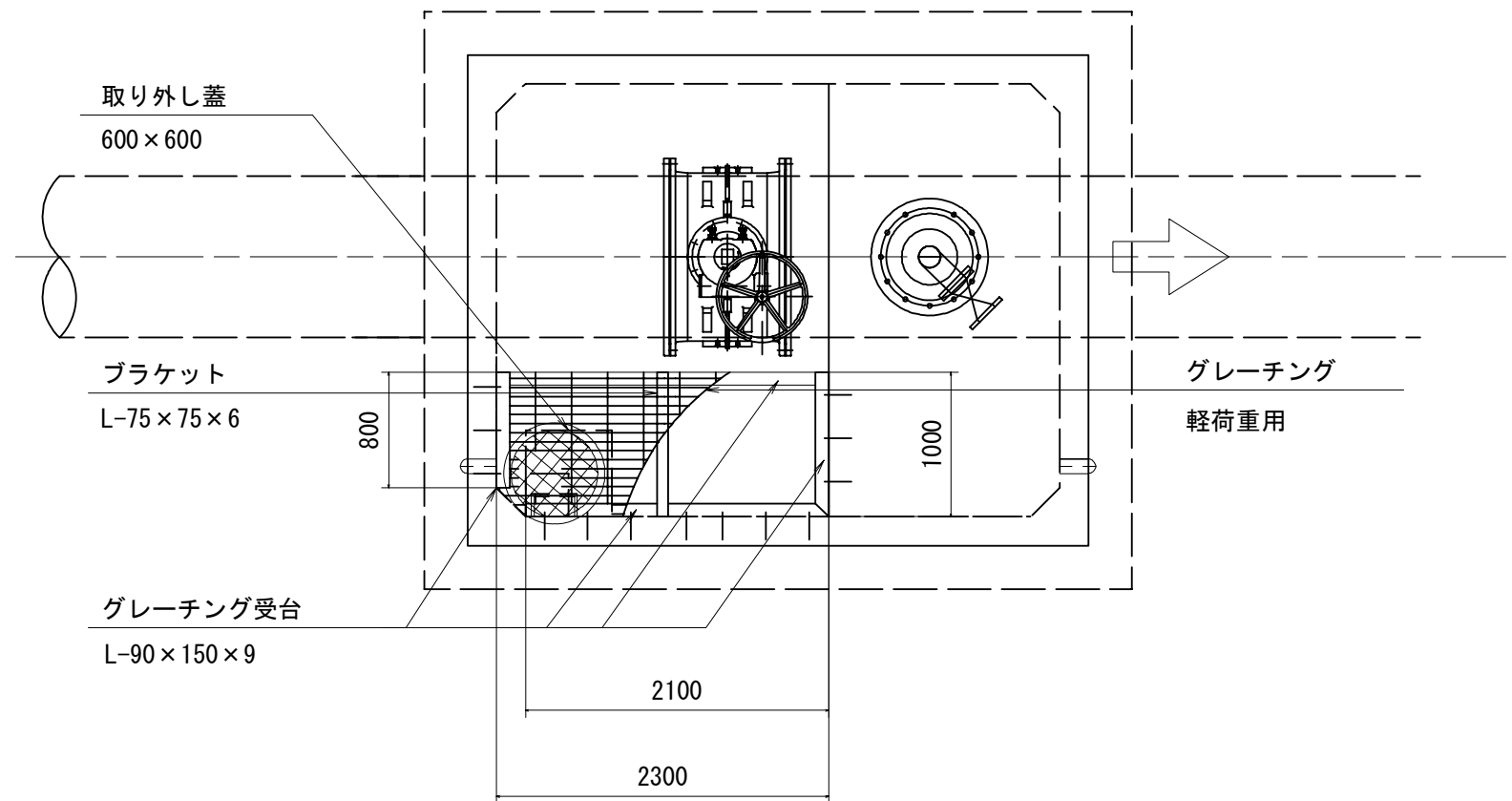
平面図
